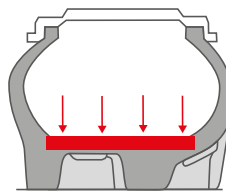
Radialkarkasse
